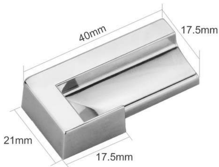
AS101E-L END CAP
